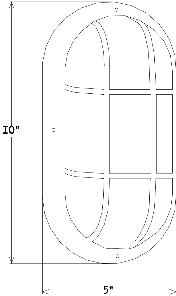
LED13 (Array)
